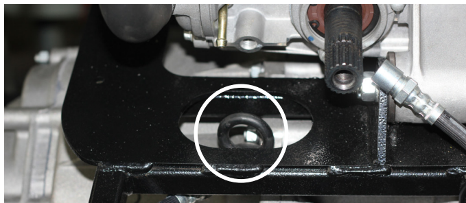
Рис. 6.2.1. Расположение контрольного щупа коробки передач
