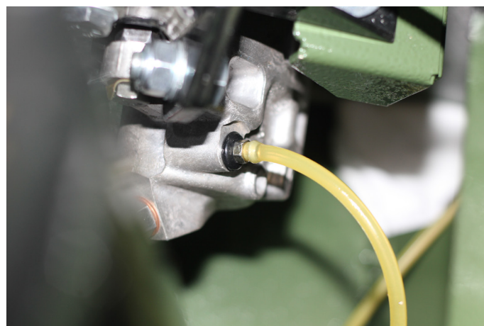
Рис. 7.3.3.1 Прокачный штуцер на суппорте тормоза
