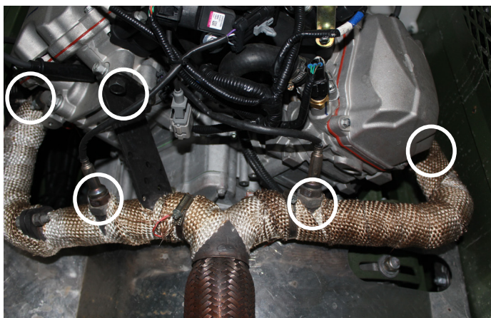
Рис. 7.9.1 Места крепления выпускного коллектора к двигателю вездехода
