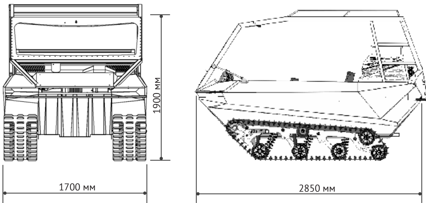
Рис. 1.4.1. Пелец Ровер III (габариты)
