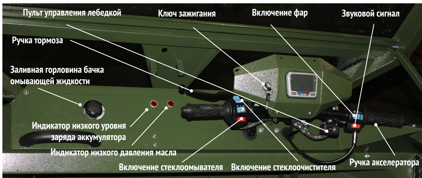
Рис. 1.6.1 Элементы управления движением вездехода
