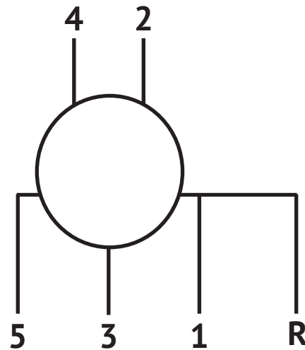
Рис. 1.6.4 Схема переключения передач
