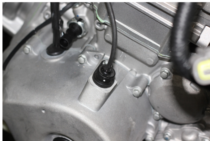
Рис. 6.5.1 Расположение датчика положения коленчатого вала
