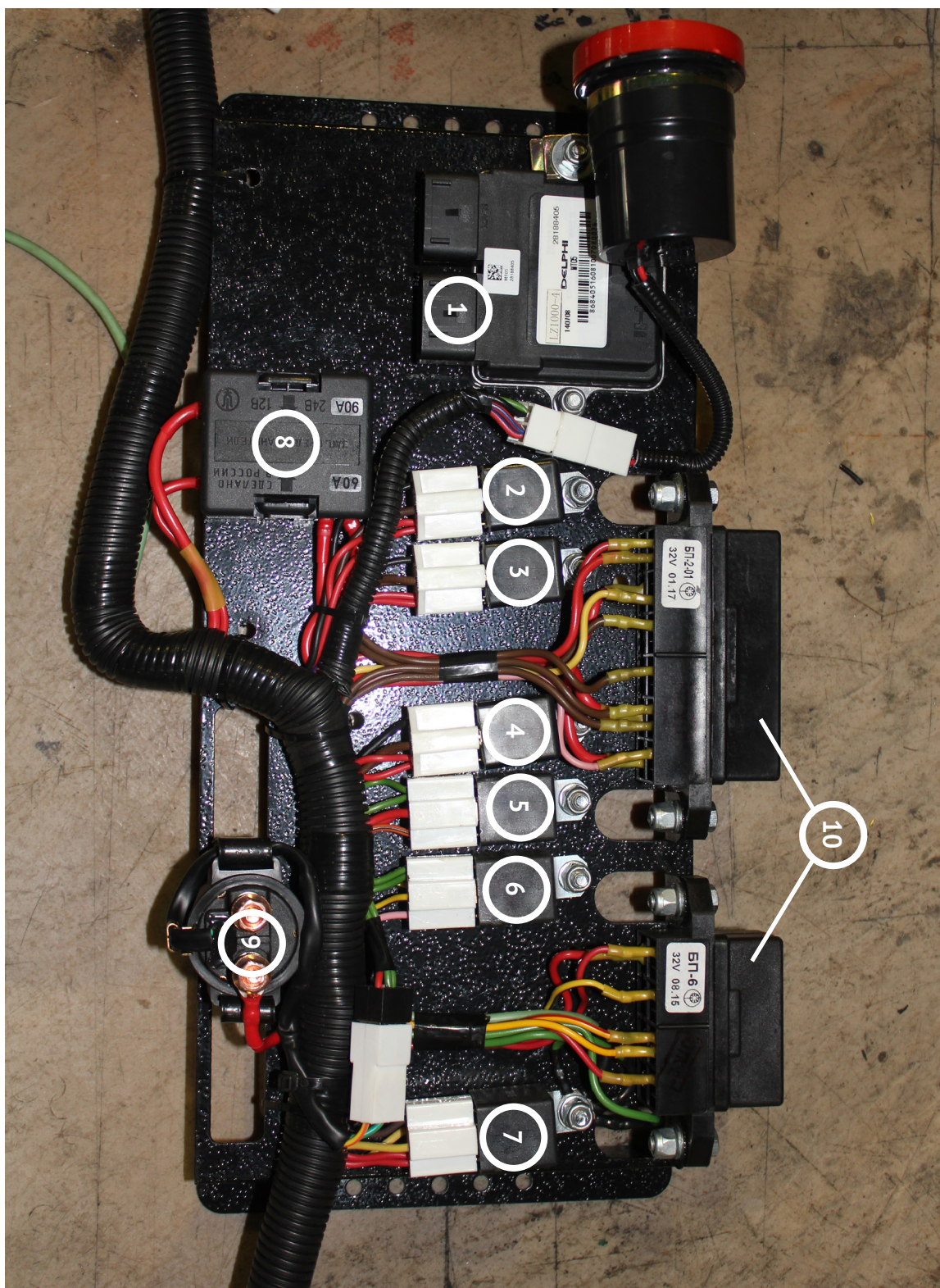
Рис. 6.7. Реле и предохранители. 1 - ББУ, 2 - реле первого вентилятора, 3 - реле второго вентилятора, 4 - реле третьего вентилятора, 5 - мастер-реле, 6 - реле дворника, 7 - реле бензобака, 8 - предохранители генераторов, 9 - реле стартера, 10 - тугоплавкие предохранители.
