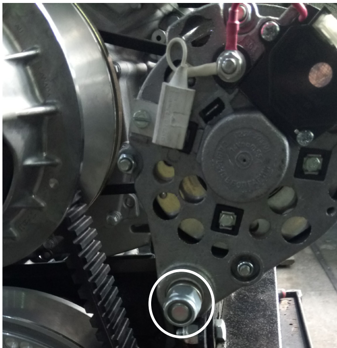
Рис. 7.9.6 Фиксирующий болт генератора
