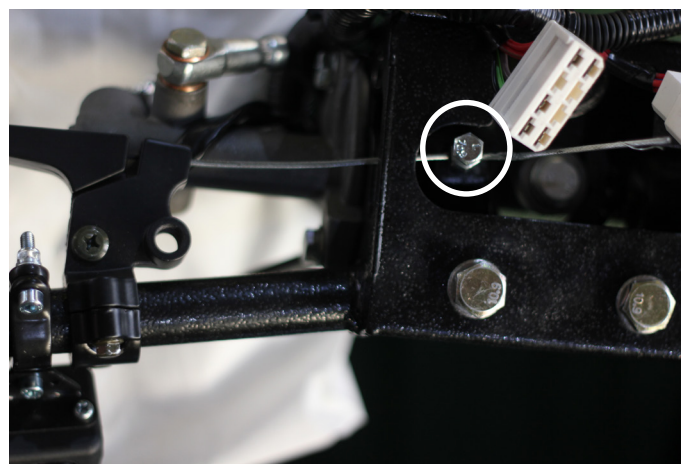
Рис. 7.8. Расположение фиксирующего болта тормозного тросика
